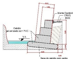
CORTE TÍPICO DO GABIÃO
