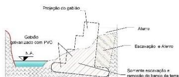
CORTE TÍPICO DO TERRENO
